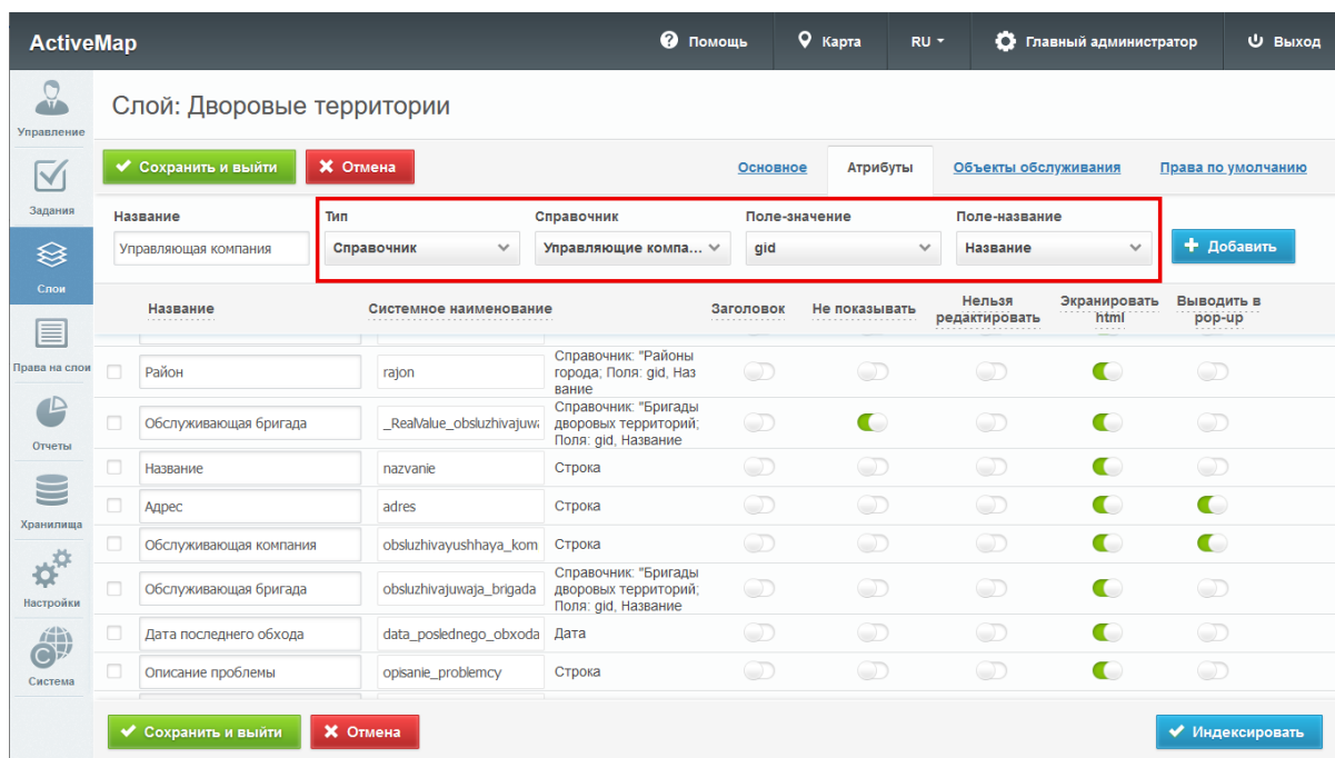
Рис. 2.74: Прикрепление справочника к полю слоя
