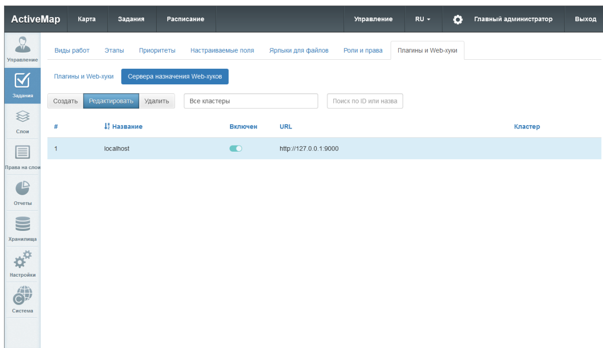
Рис. 2.65: Список серверов назначения Web-хуков
