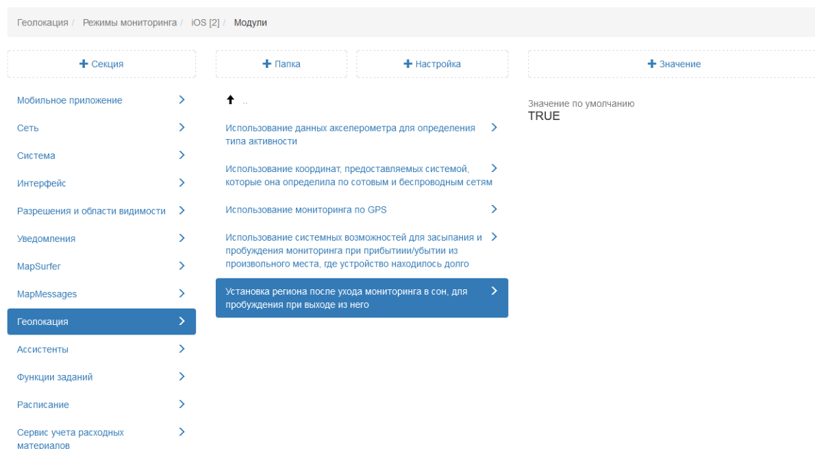
Рис. 2.233: Установка региона после ухода мониторинга в сон, для пробуждения при выходе из него
