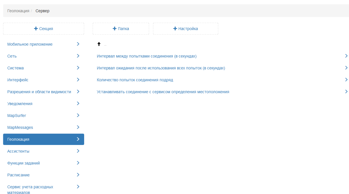
Рис. 2.249: Серверные настройки мониторинга геолокации
