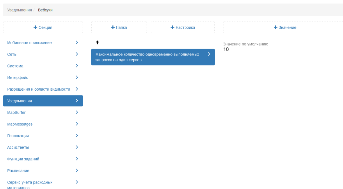
Рис. 2.191: Максимальное количество одновременно выполняемых запросов на один сервер
