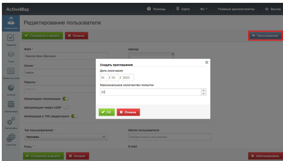
Рис. 2.41: Создание приглашения из карточки пользователя
