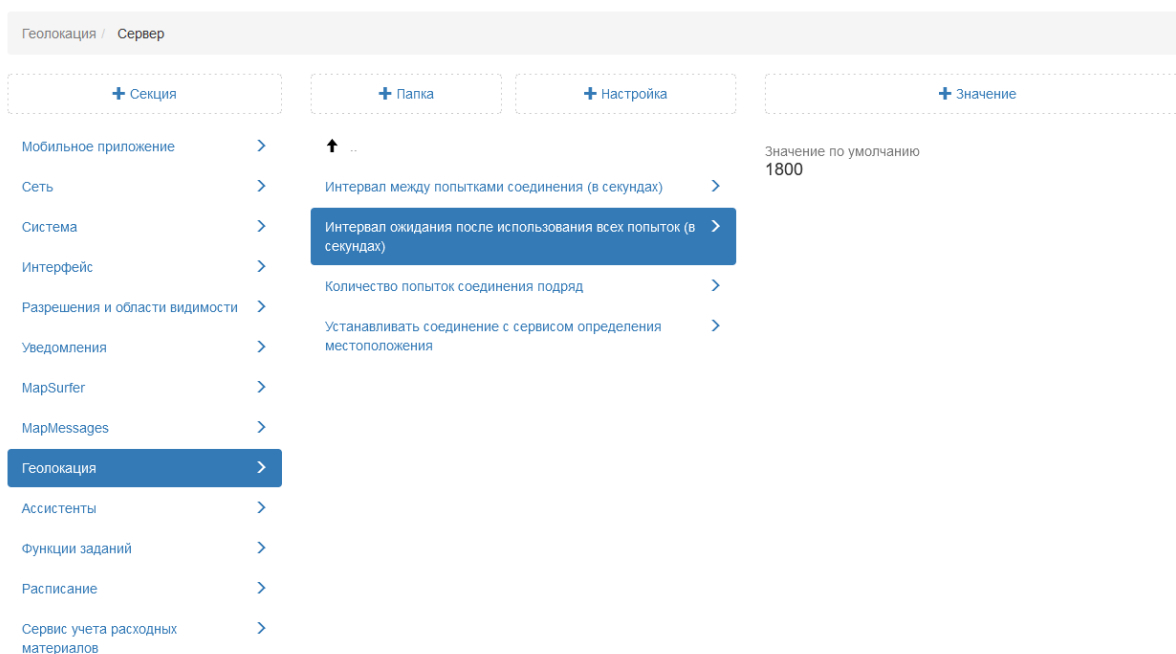
Рис. 2.253: Интервал ожидания после использования всех попыток
