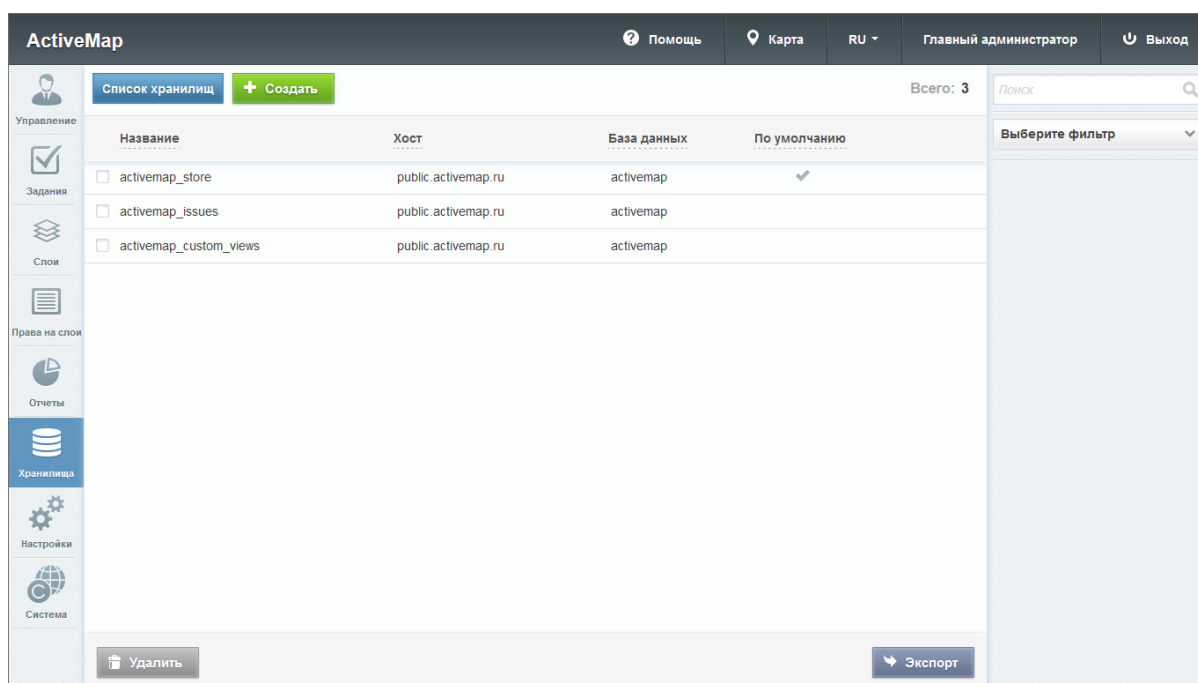
Рис. 2.105: Блок «Хранилища»
