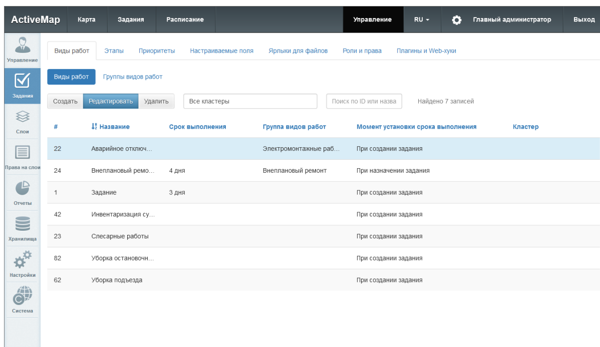
Рис. 2.50: Блок «Задания»
