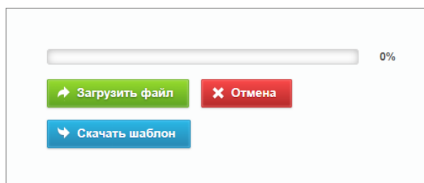
Рис. 2.30: Импорт пользователей
