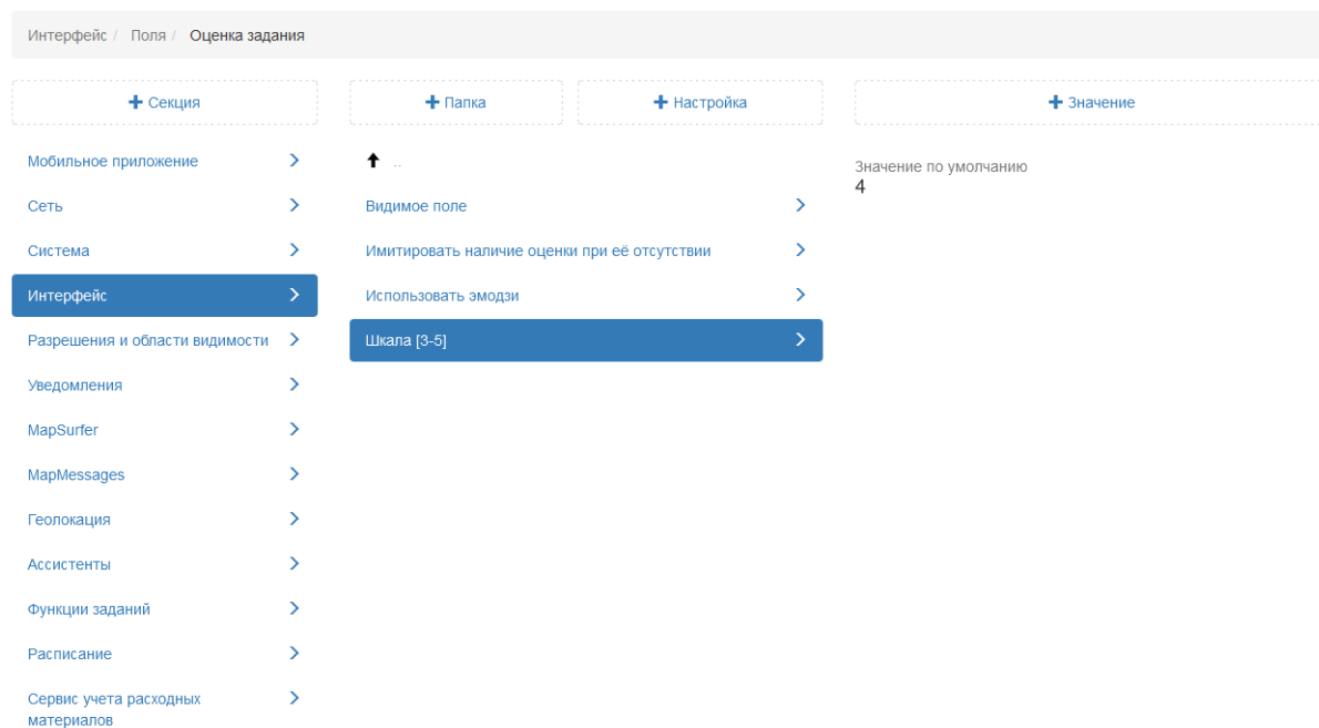
Рис. 2.183: Использование эмодзи
