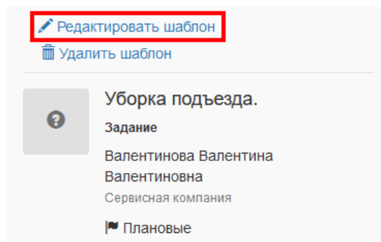
Рис. 2.24: Редактирование шаблона
