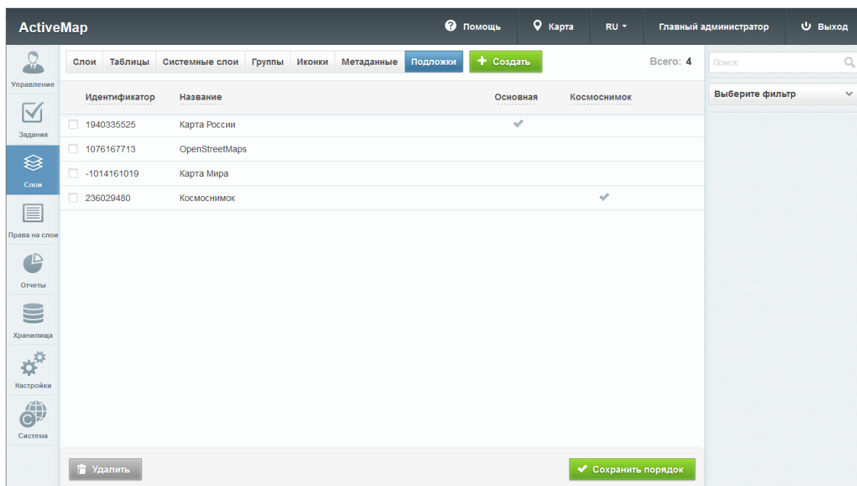
Рис. 2.94: Вкладка «Подложки»
