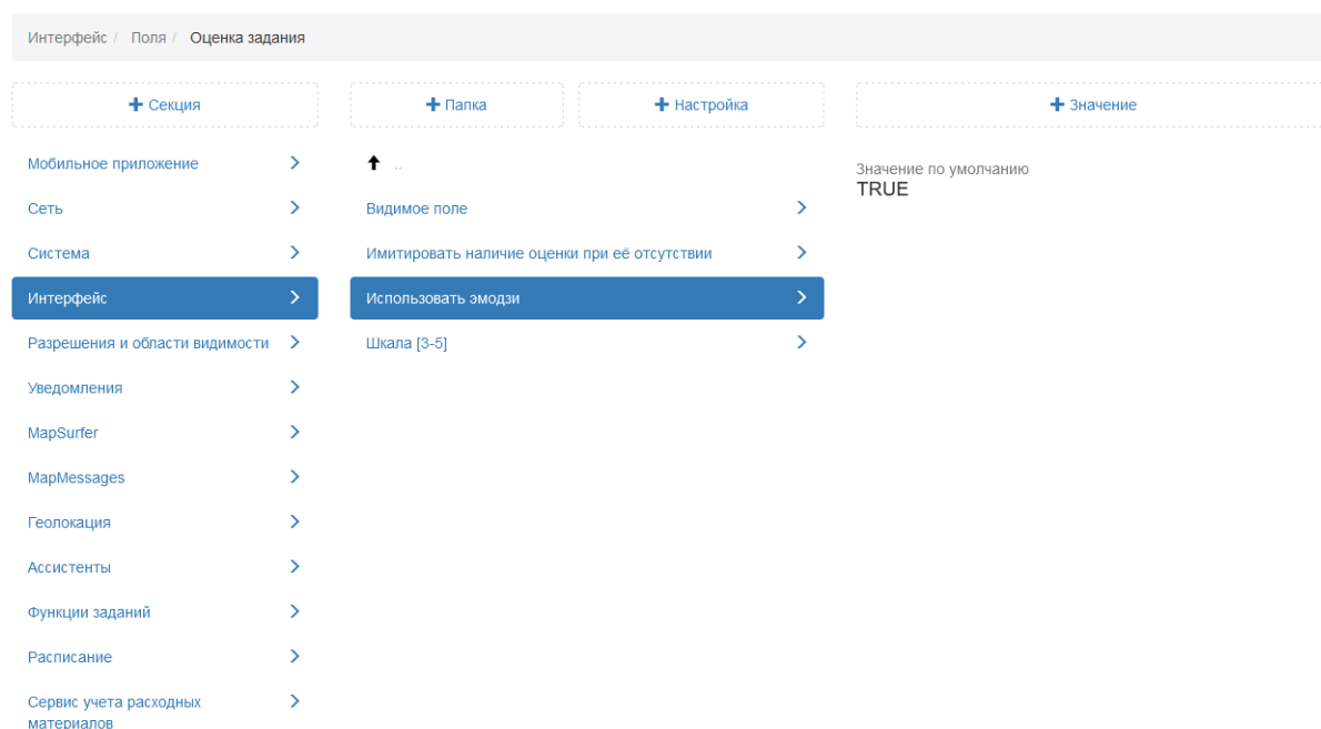
Рис. 2.182: Использование эмодзи
