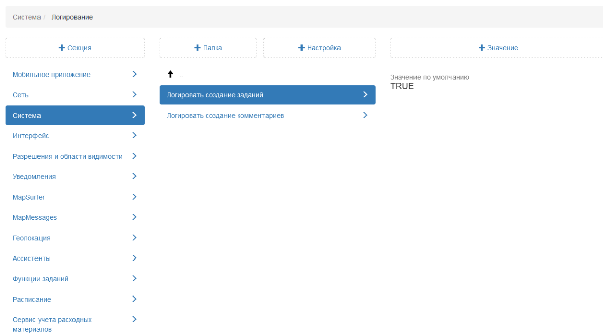
Рис. 2.179: Логирование
