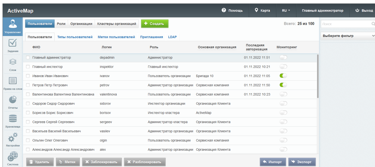
Рис. 2.29: Вкладка «Пользователи»
