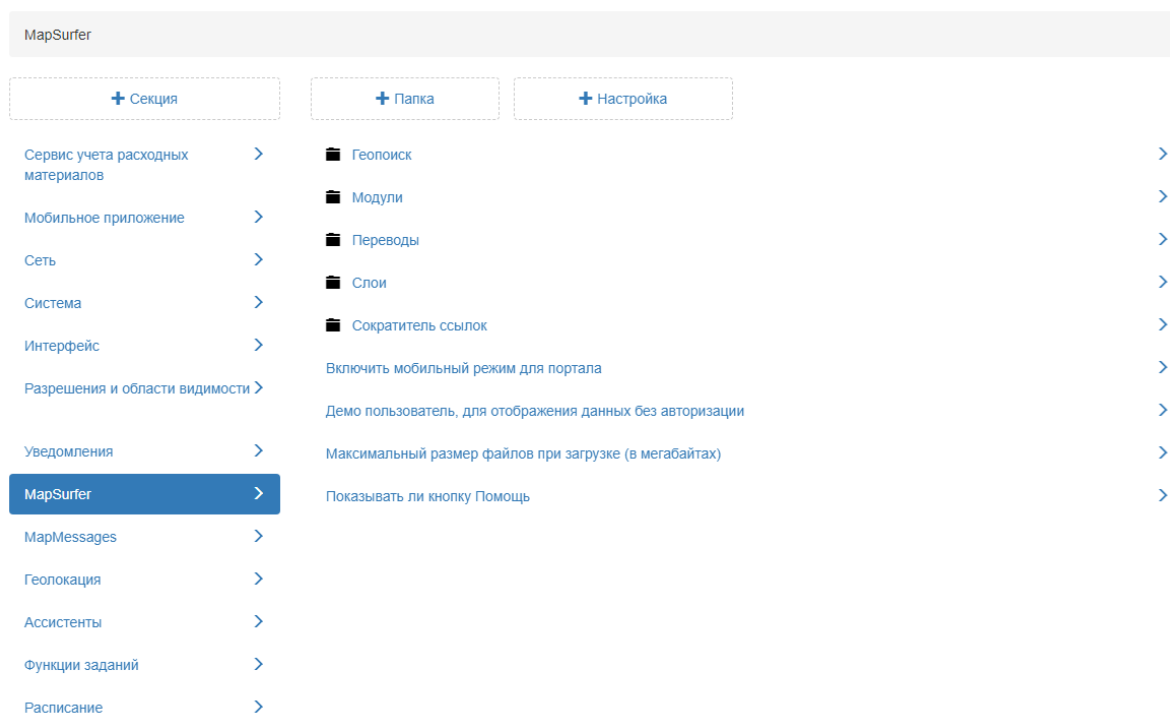
Рис. 2.192: Секция «MapSurfer»
