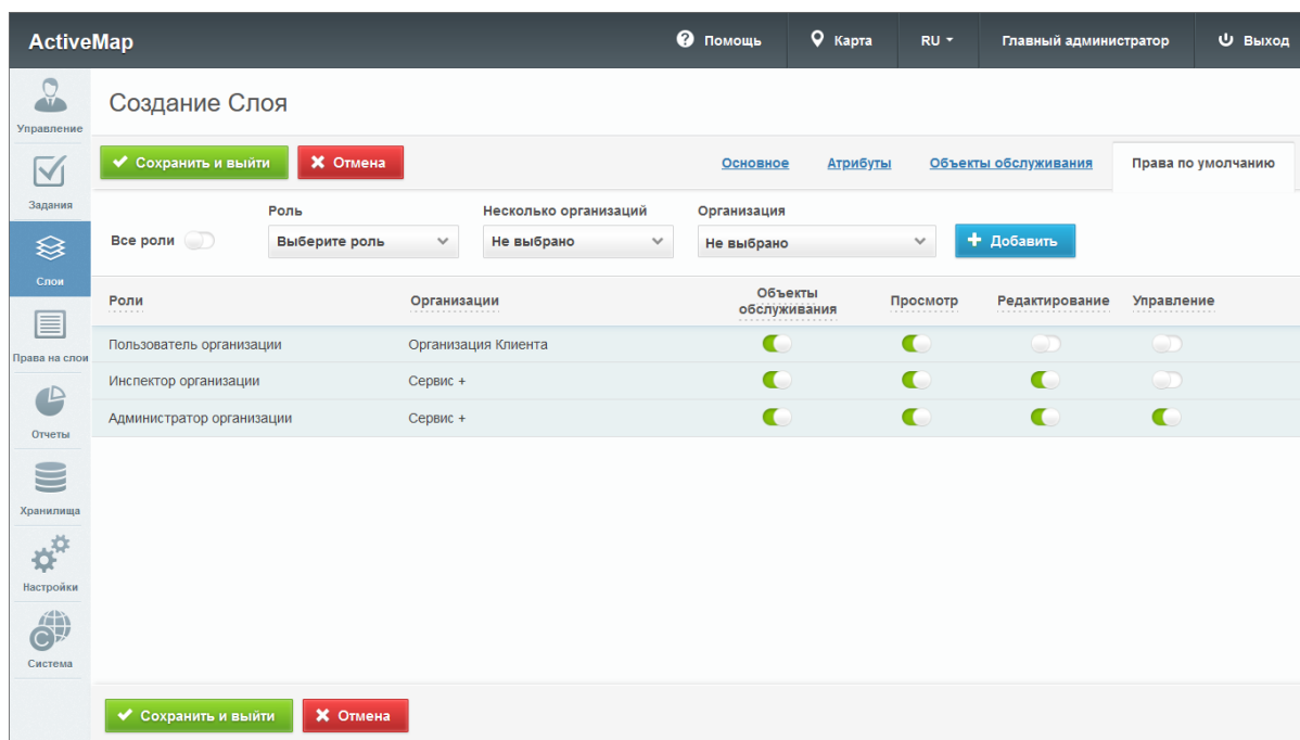
Рис. 2.77: Вкладка «Права по умолчанию»
