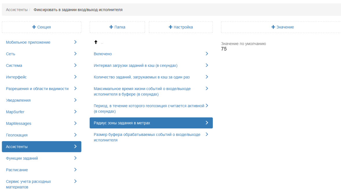
Рис. 2.266: Радиус зоны задания
