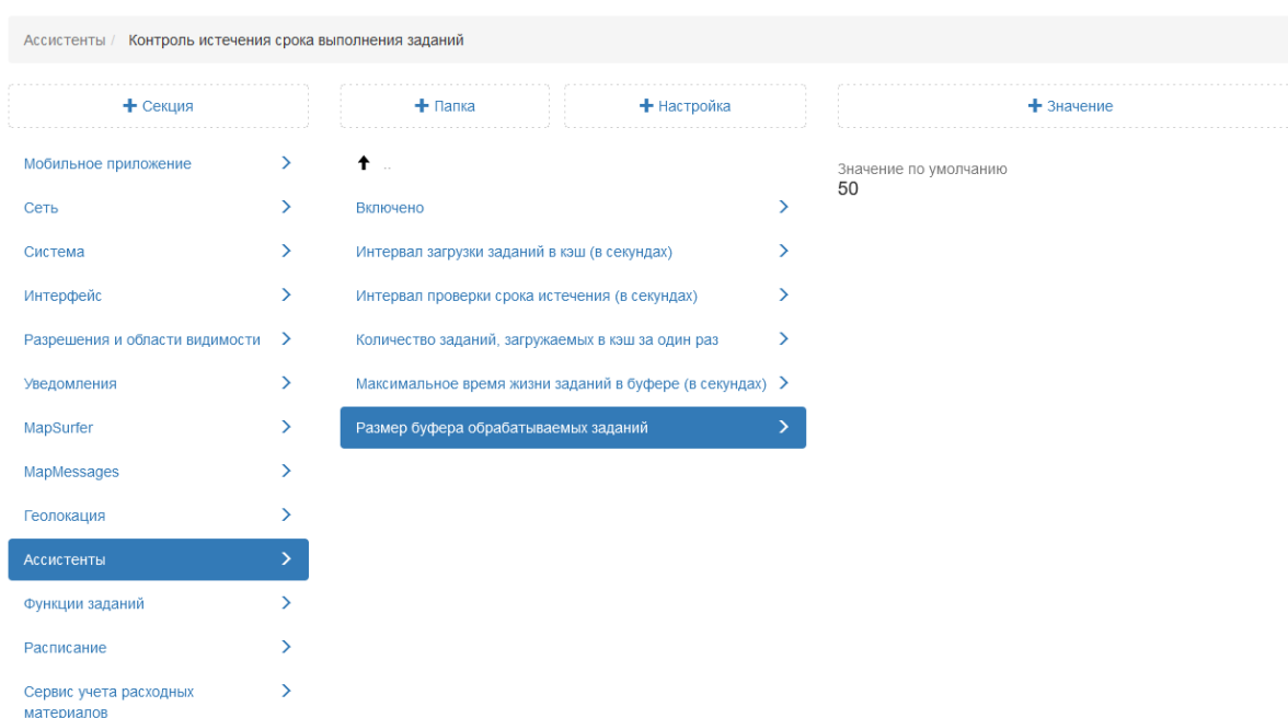
Рис. 2.263: Размер буфера обрабатываемых заданий
