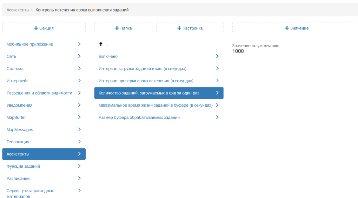
Рис. 2.260: Количество заданий, загружаемых в кэш за один раз
