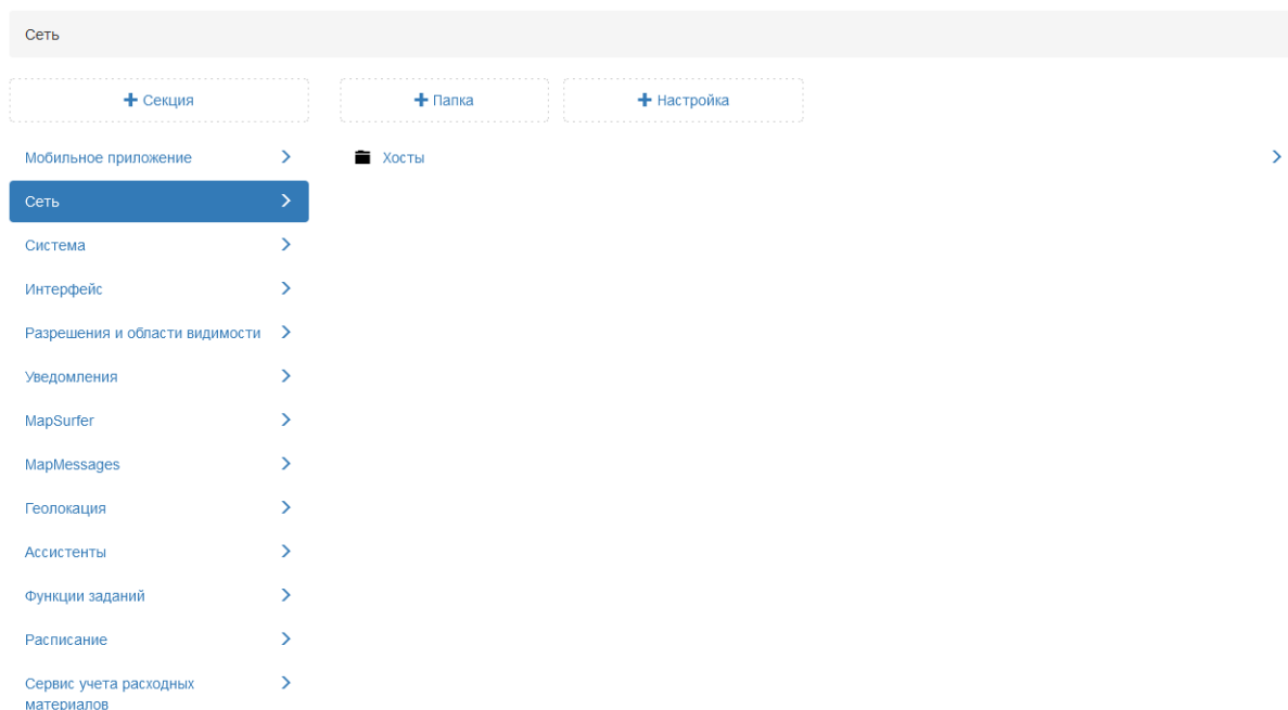
Рис. 2.155: Секция «Сеть»
