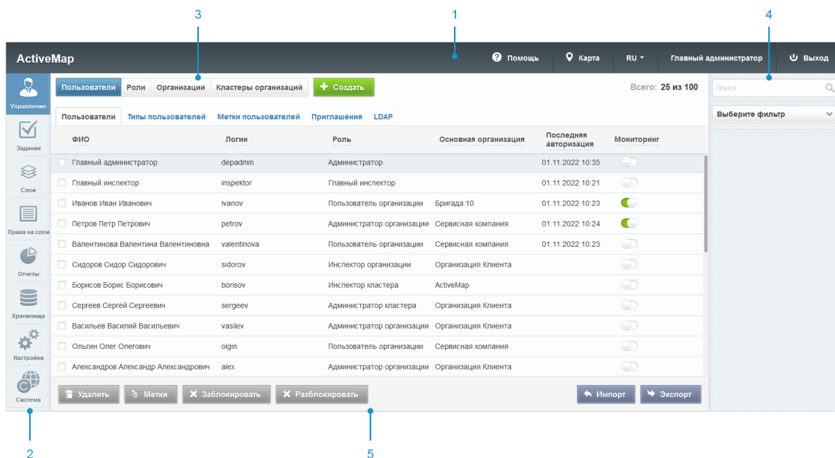
Рис. 2.27: Модуль управления
