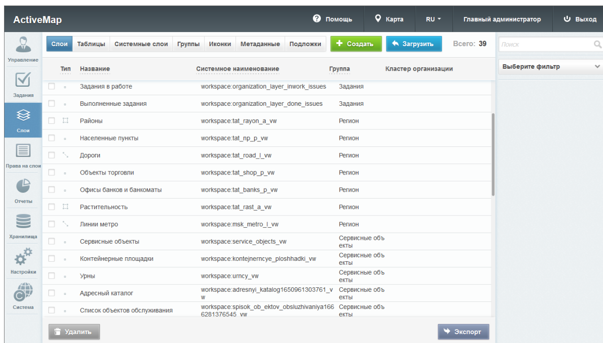
Рис. 2.66: Блок «Слои»
