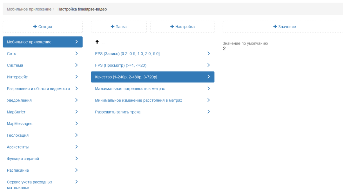
Рис. 2.145: Качество
