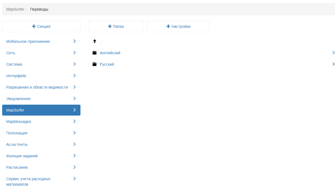
Рис. 2.203: Переводы
