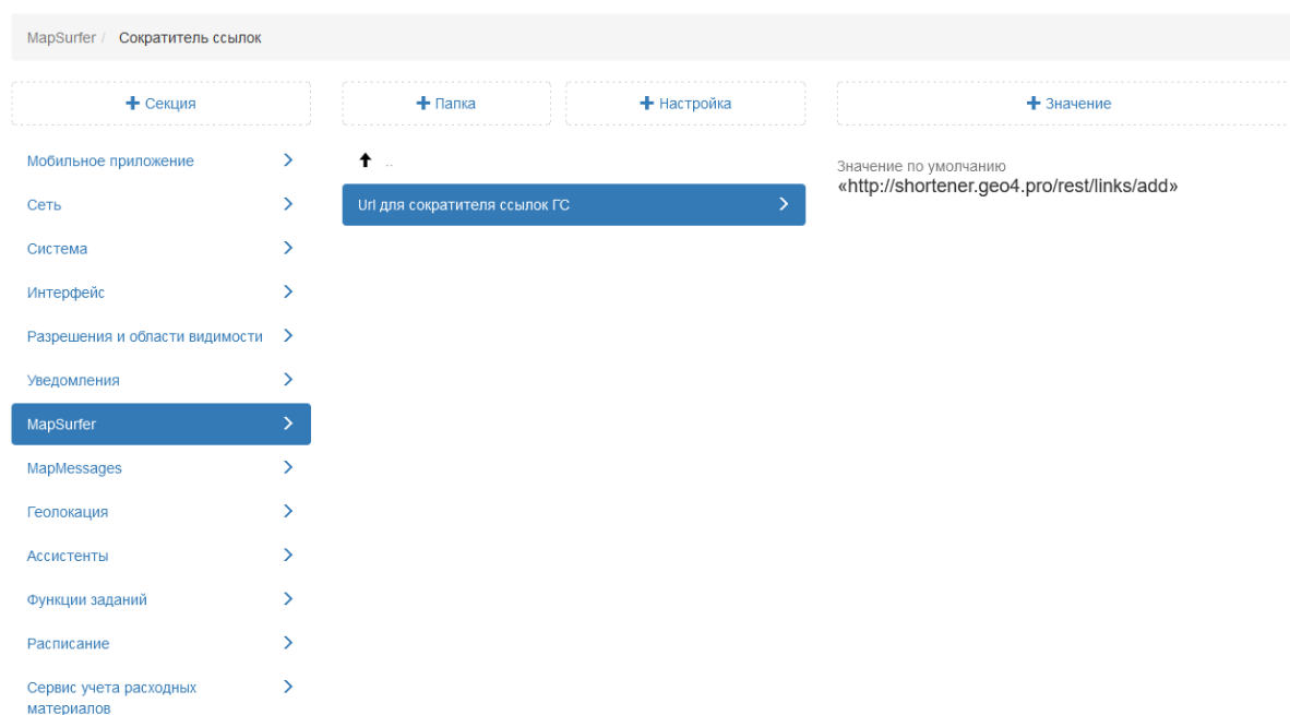
Рис. 2.215: Сократитель ссылок
