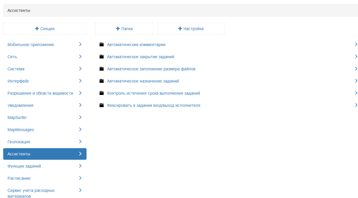
Рис. 2.254: Секция «Ассистенты»
