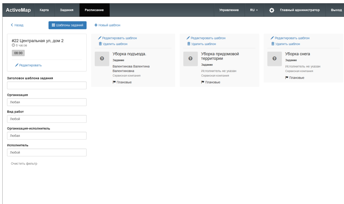
Рис. 2.22: Шаблоны заданий
