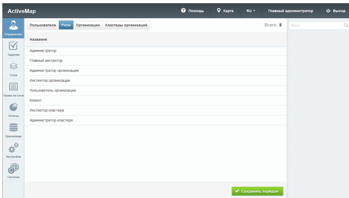
Рис. 2.43: Вкладка «Роли»
