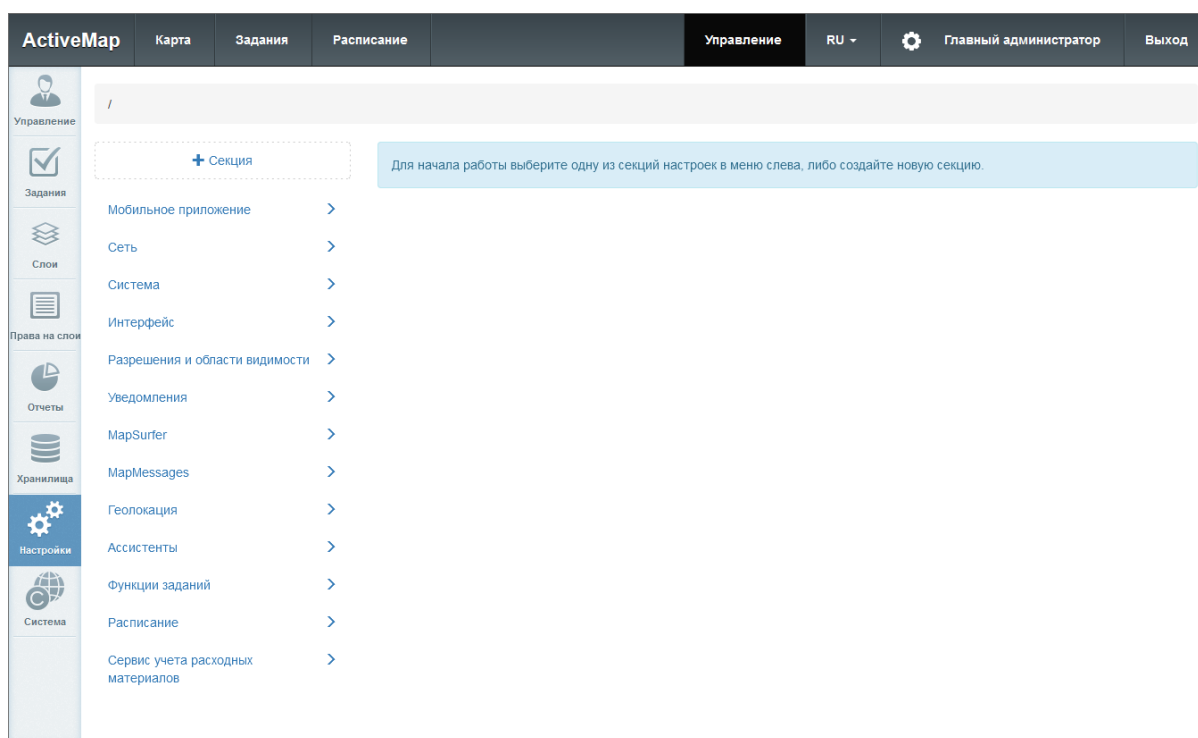
Рис. 2.108: Блок «Настройки»
