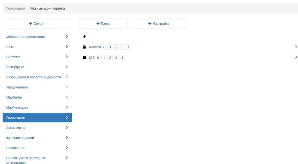
Рис. 2.228: Режимы мониторинга
