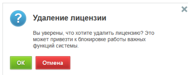
Рис. 2.284: Подтверждение удаления
