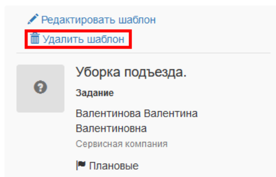
Рис. 2.25: Удаление шаблона
