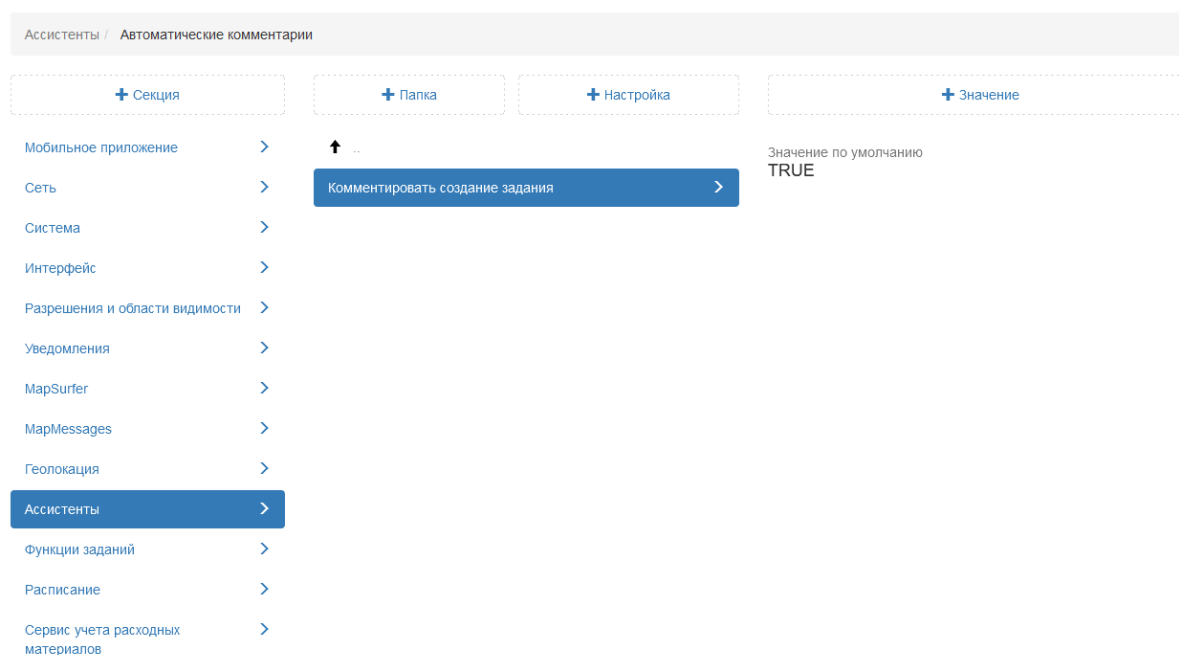
Рис. 2.255: Автоматические комментарии
