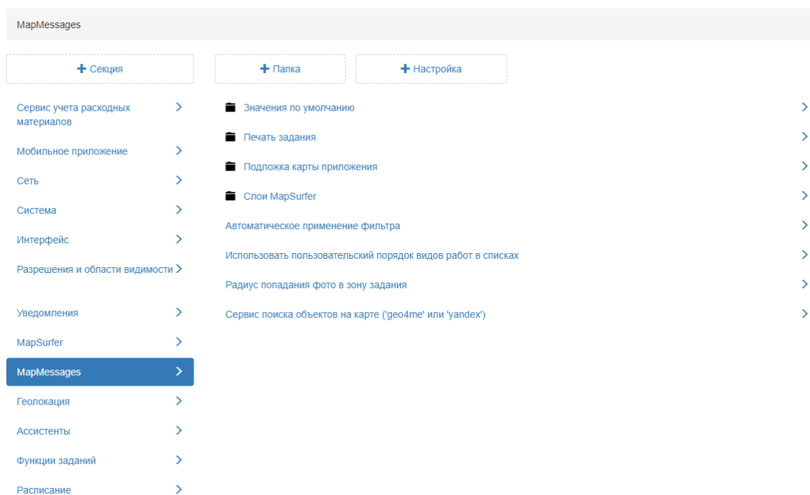
Рис. 2.220: Секция «MapMessages»
