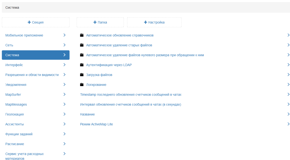
Рис. 2.160: Секция «Система»
