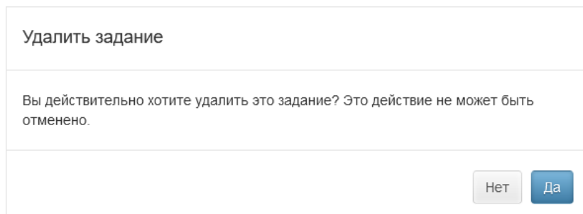
Рис. 2.14: Удаление задания
