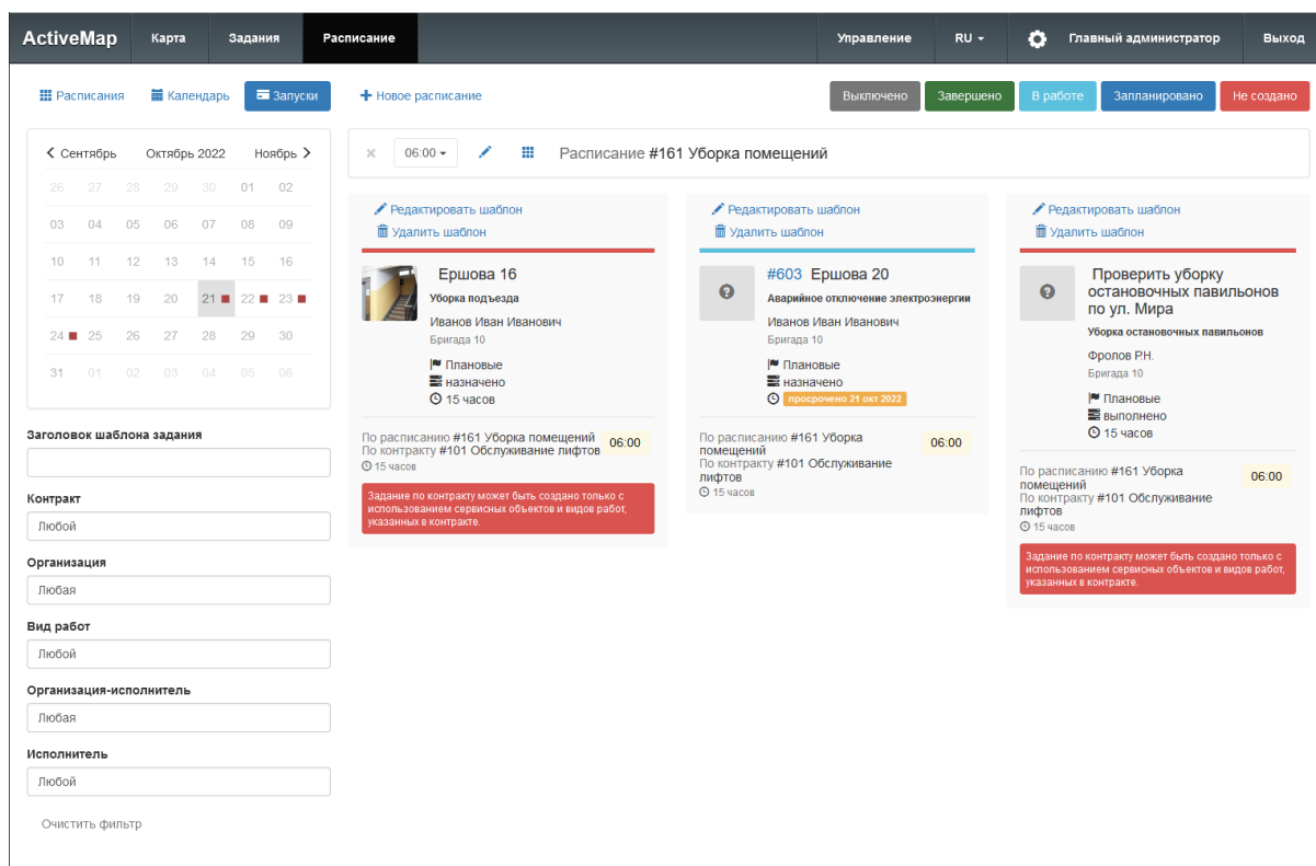
Рис. 2.18: Шаблоны заданий
